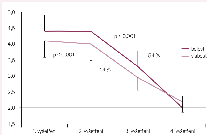
Graf 1. Změny subjektivních pocitů.
