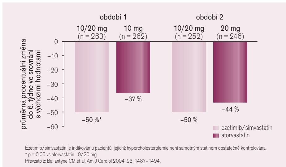
Graf 8. Výsledky studie VYVA-LDL-C.
